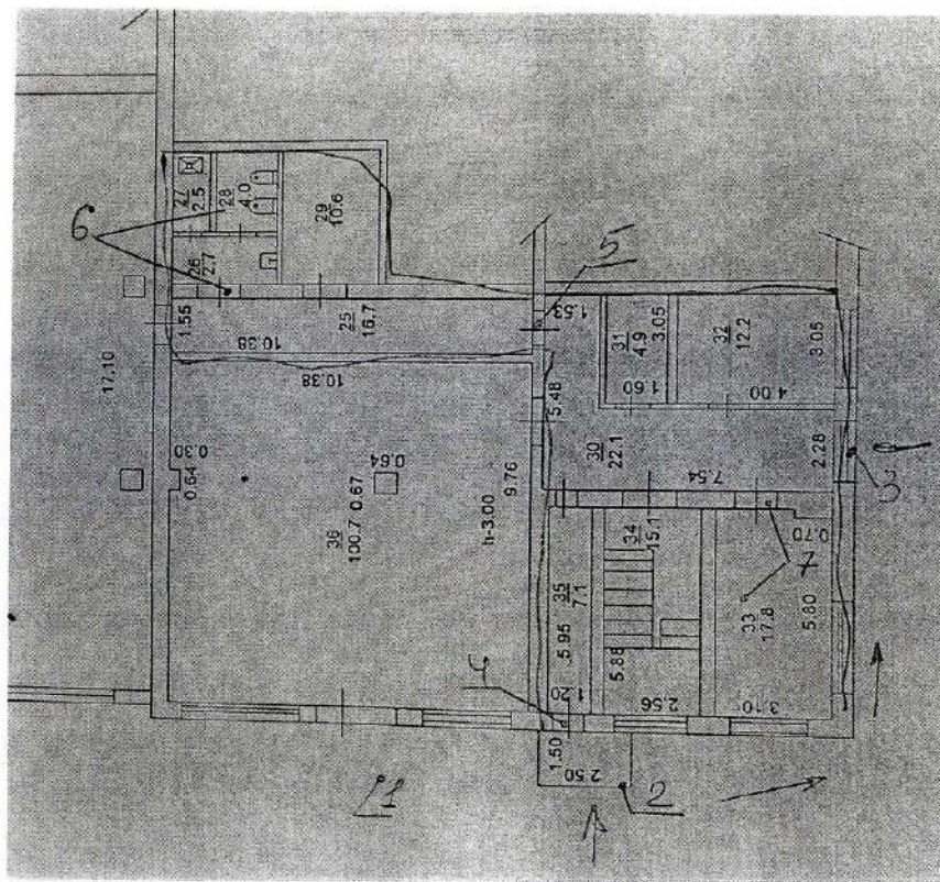
План-Схема здания учебного полигона ГБОУ СПО РО «РАДК», г.Ростов-на-Дону, ул. Вавилова, 80
